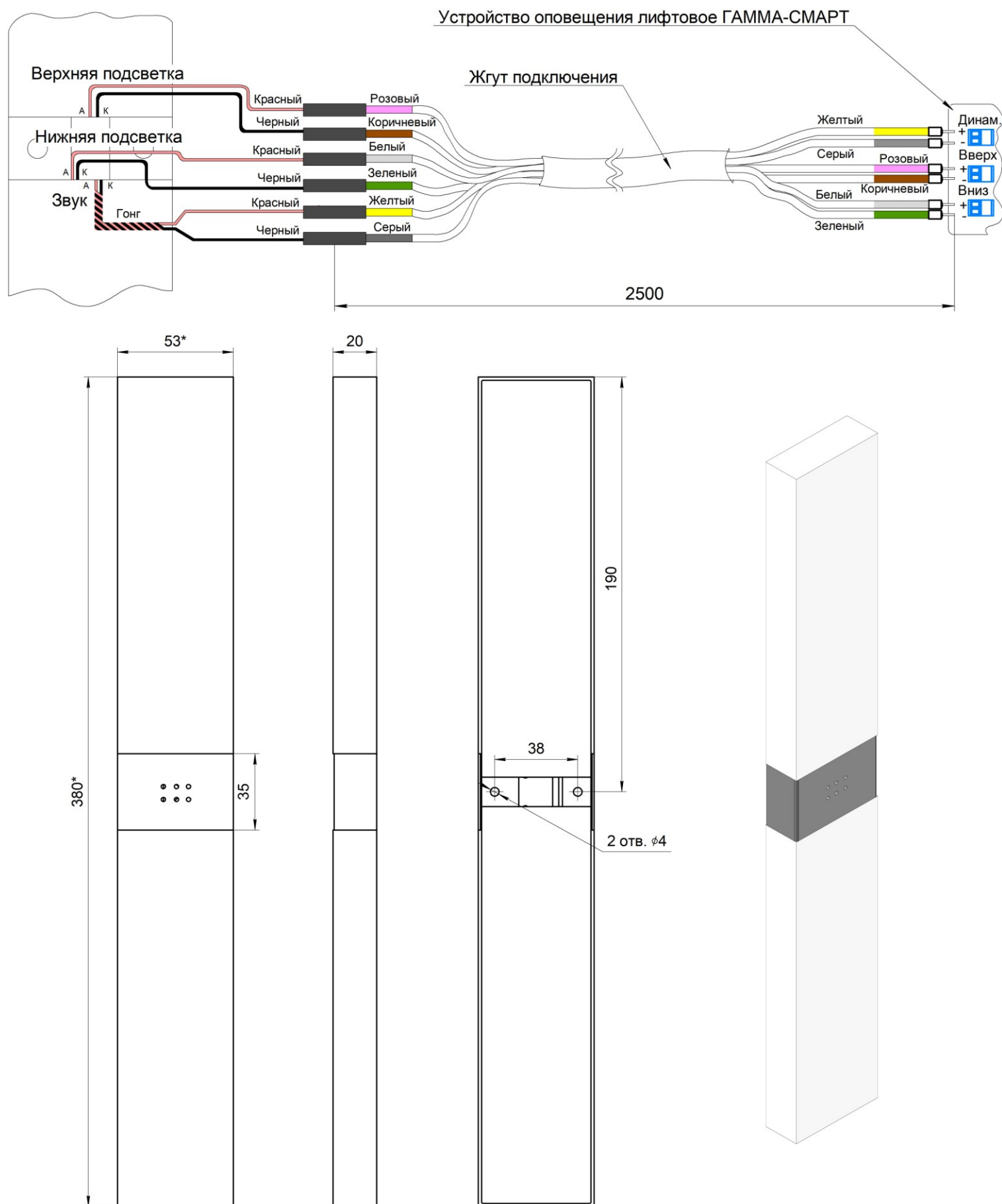
Рис.1 Внешний вид «Указатель лифтовой» НШЕК.468232.200
